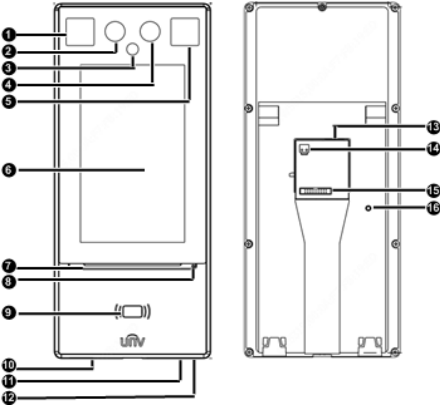
图3-2 设备结构图
